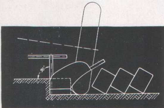
Richtige Querneigung beim Arbeiten in der Ebene
