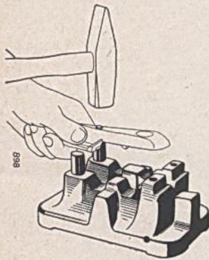
Vernieten der Fingerplatte.
