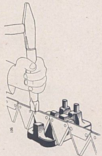
Abnieten der nicht überstehenden Messerklinge.
