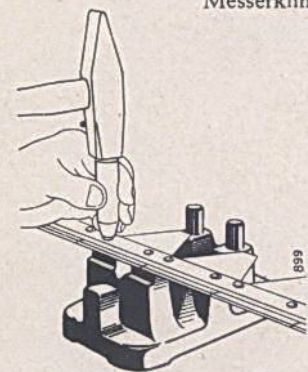
Aufnieten der Messerklinge bei beiderseitigem Rundkopf.
