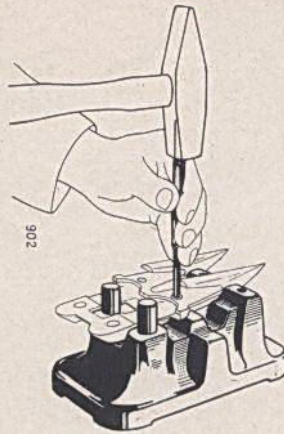
Abnieten der Fingerplatte beim Mittelschnitt-Doppelfinger.
