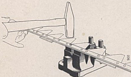
Aufnieten der Klinge auf den Messerrücken.
