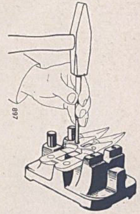
Abnieten der Fingerplatte beim Tiefschnitt-Doppelfinger.
