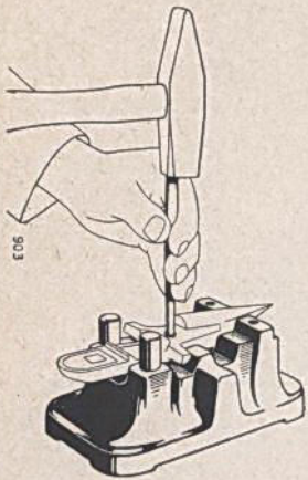
Abnieten der Fingerplatte beim Normalschnittfinger.
